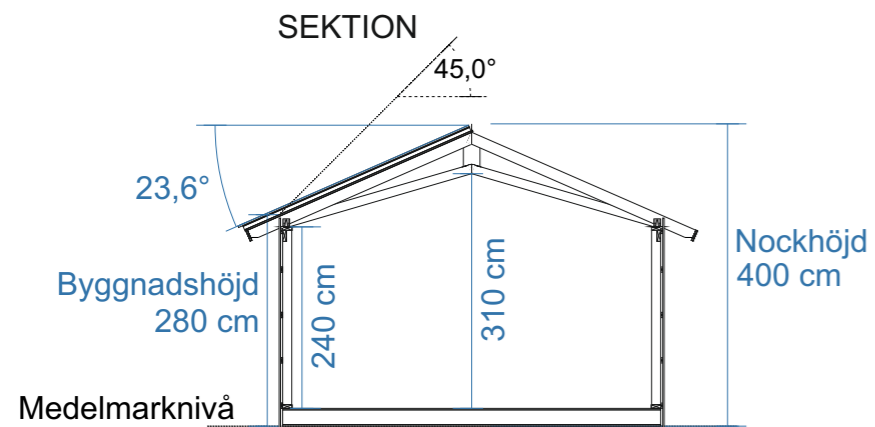
SEKTION
